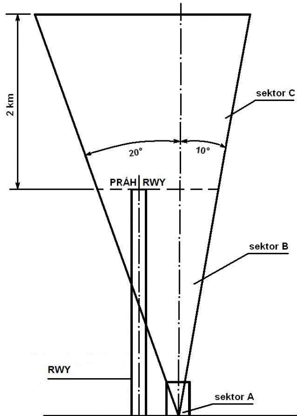
Obr. 11-7 Znáromění ochranného pásma přesného přibližovacího radaru PAR
