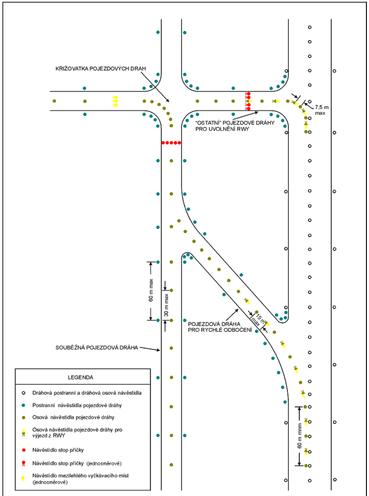
Obr. 5 - 22 Návěstidla na pojezdové dráze
