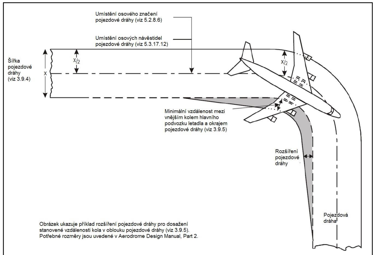
Obr. 3-2 Oblouk pojezdové dráhy
