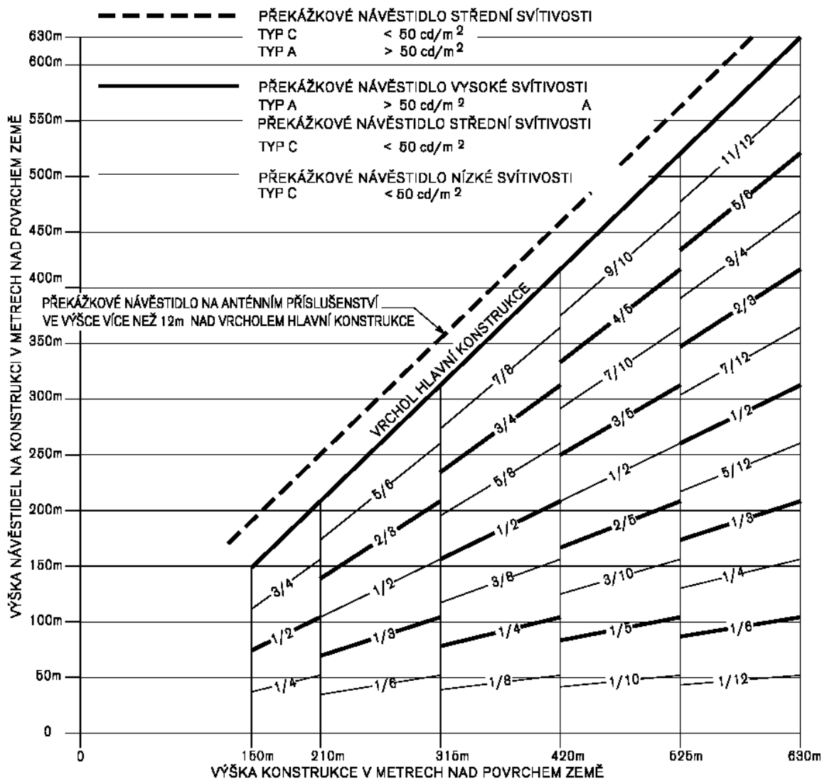
Obr. 5.8 Duální systém překážkových návěstidel vysoké a střední svítivosti typu A a typu C
