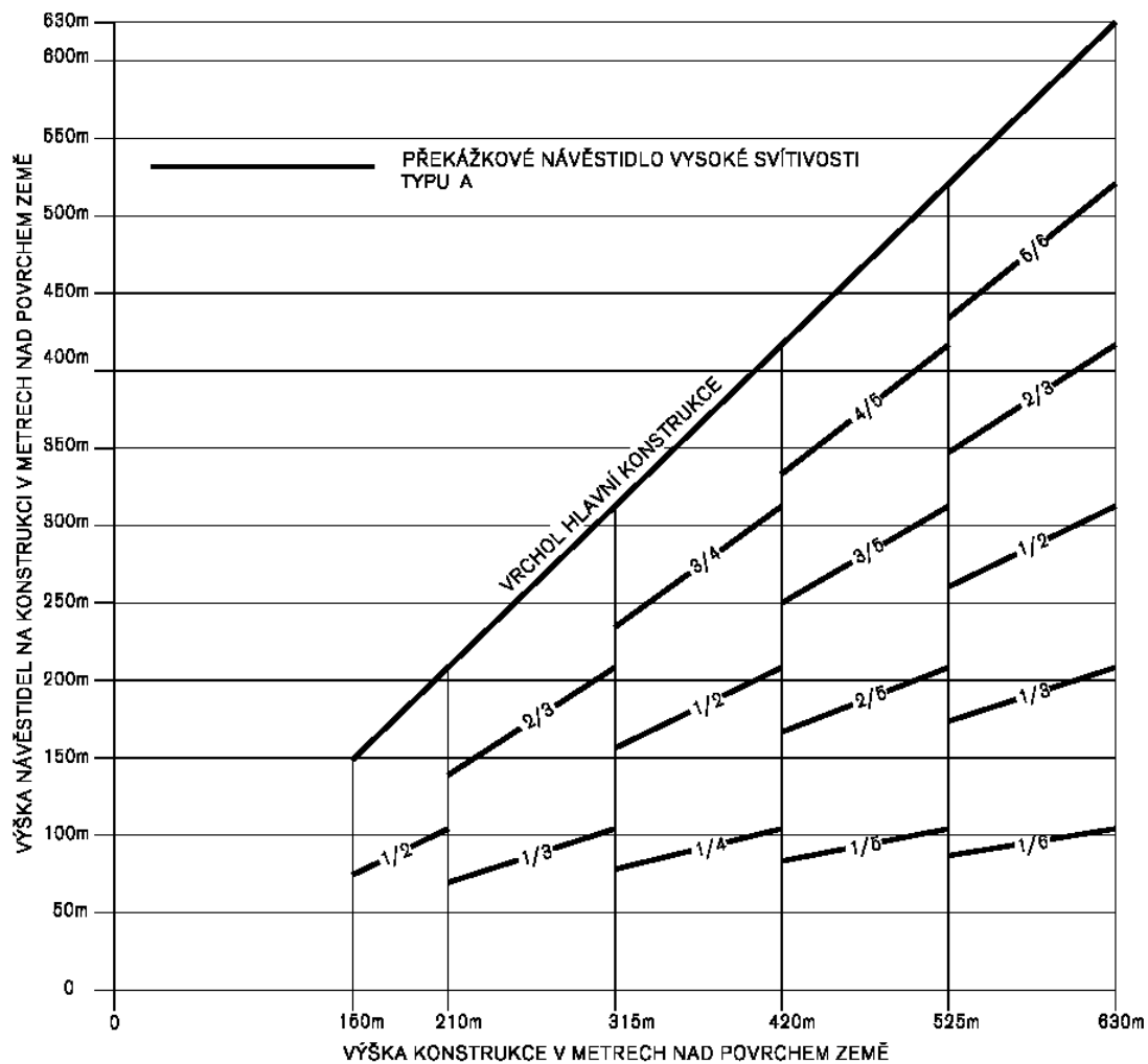
Obr. 5.6 Překážkové návěstidlo vysoké svítivosti typu A, vydávající záblesky bílé barvy
