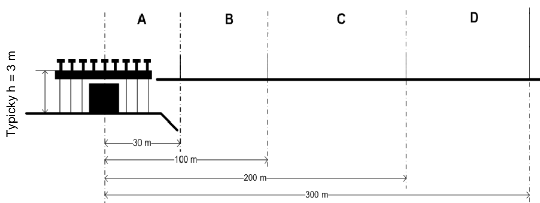
Obr. 11-11 Sektory ochranného pásma všesměrového majáku DVOR
