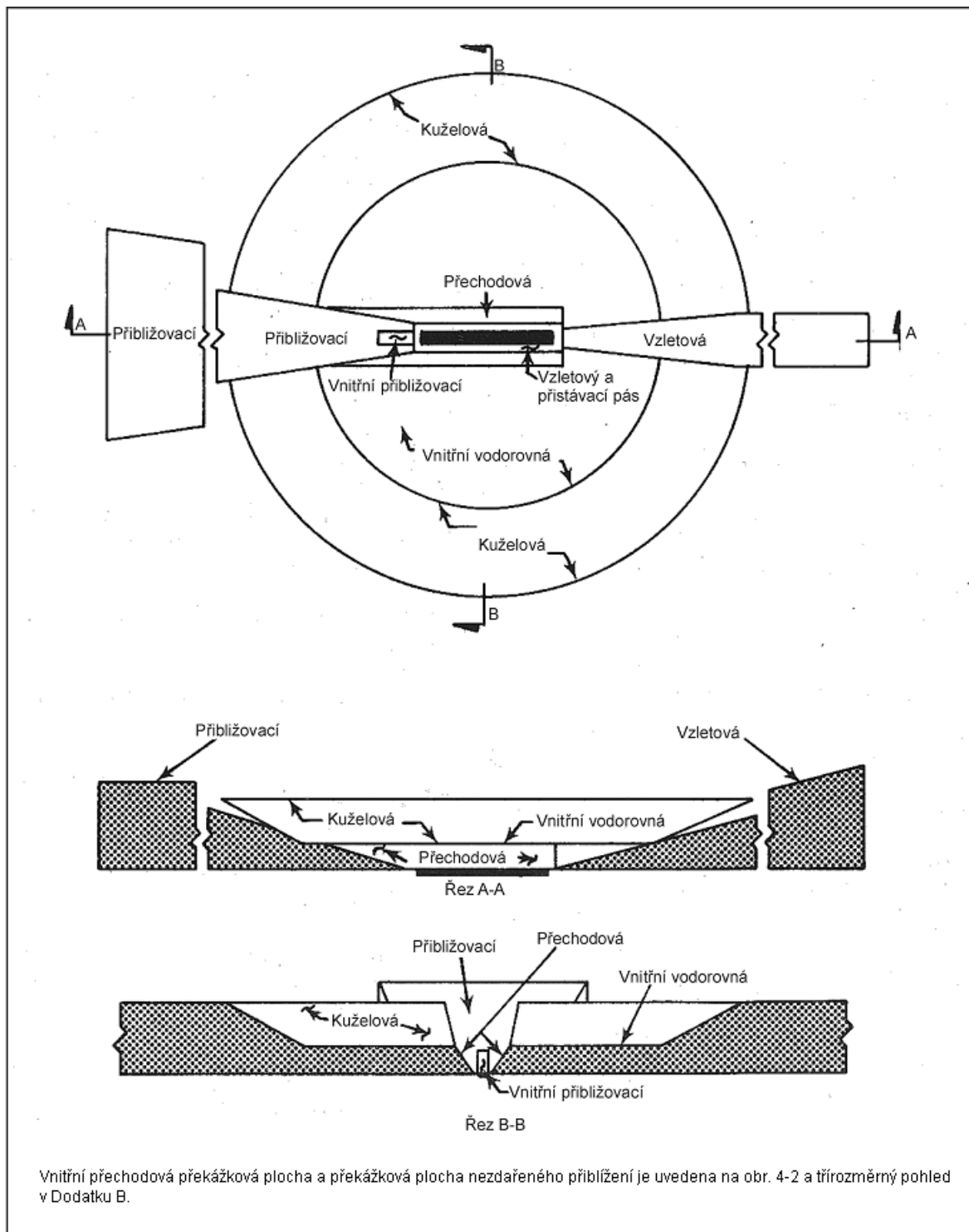
Obr. 4-1 Překážkové plochy
