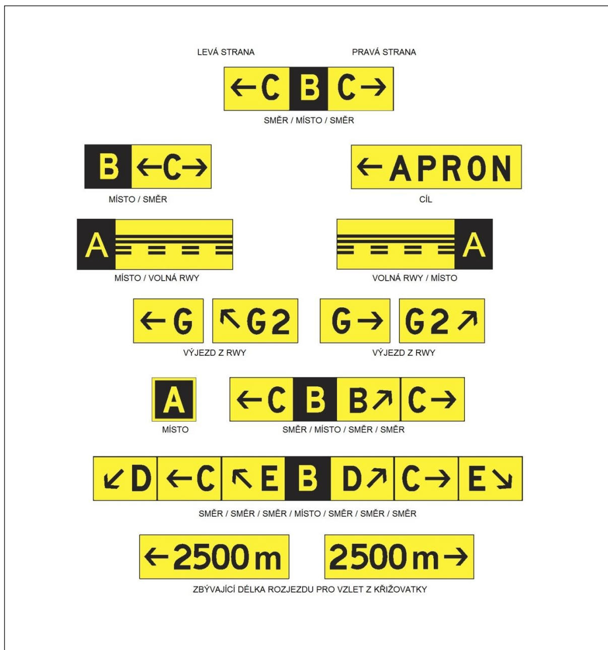
Obr. 5-28 Informační znaky
