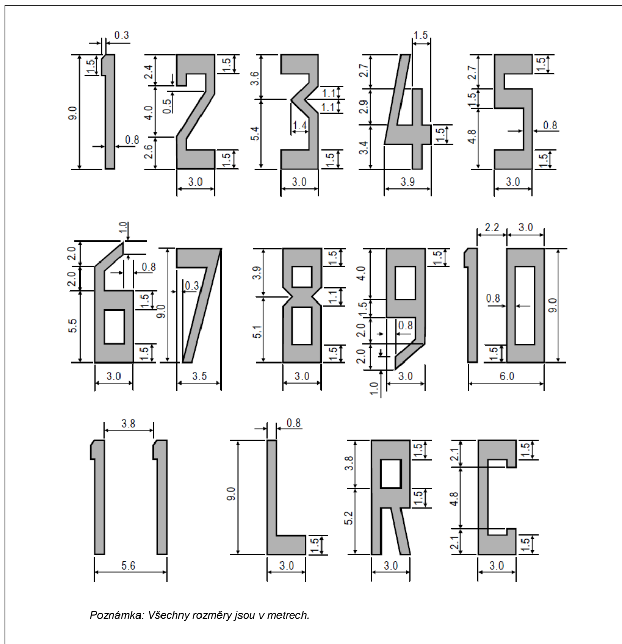
Obr. 5 - 3 Tvar a rozměry číslic a písmen dráhového poznávacího značení
