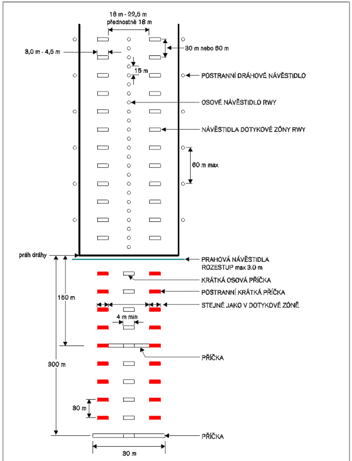
Obr. 5-11 Vnitřních 300 m světelné přibližovací a dráhové soustavy pro RWY pro přesné přiblížení II. a III. kategorie
