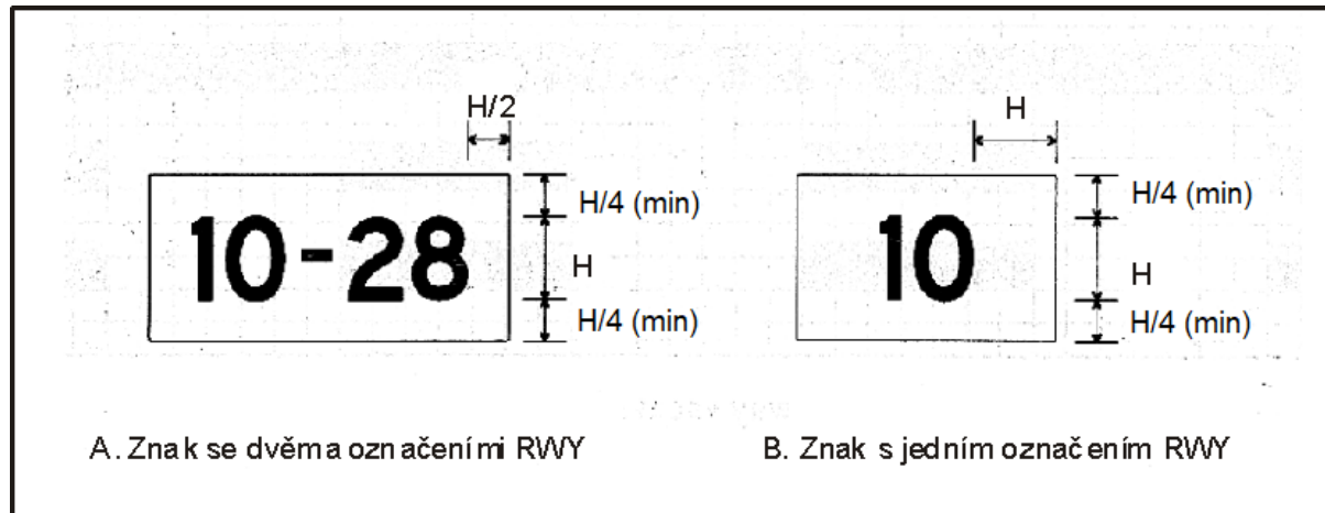
Obr. 4.4 Rozměry znaků
