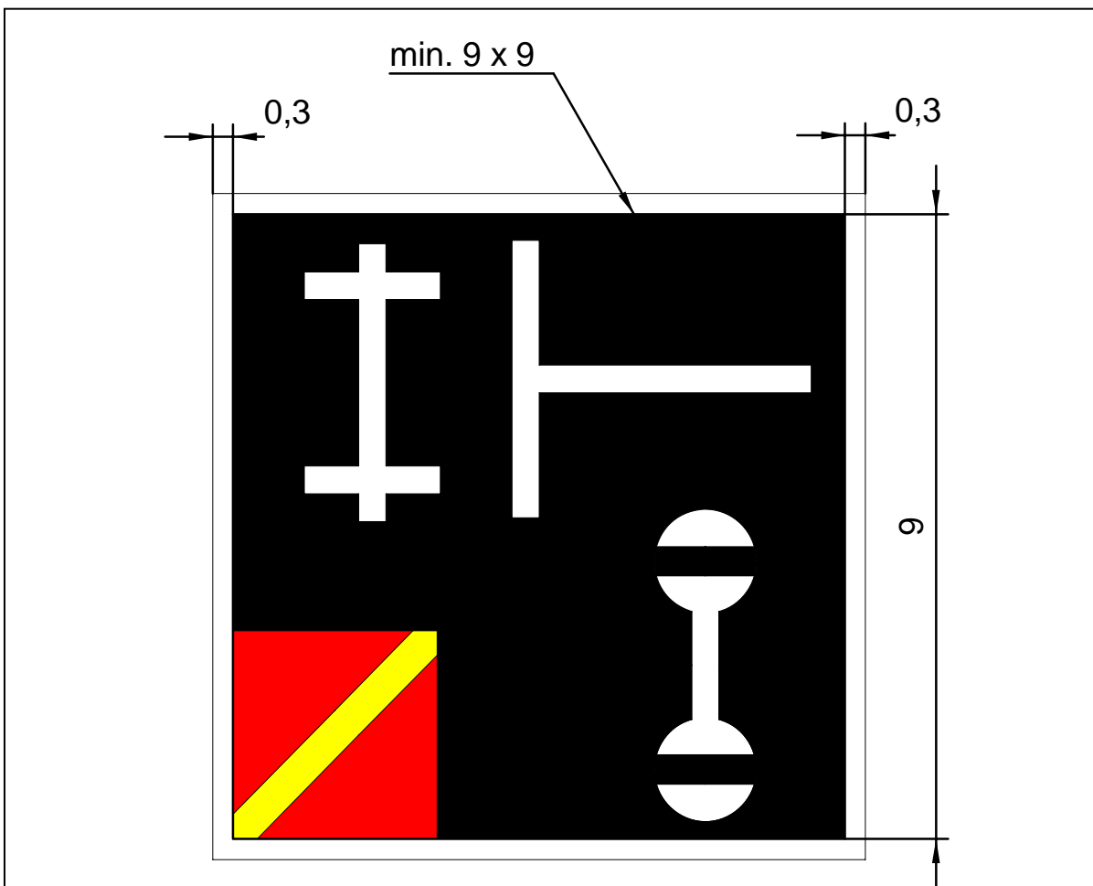
Obr. 3.9 Návěstní plocha (příklad uspořádání) (viz předpis L14, Hlava 5, ust. 5.1.4.2)
