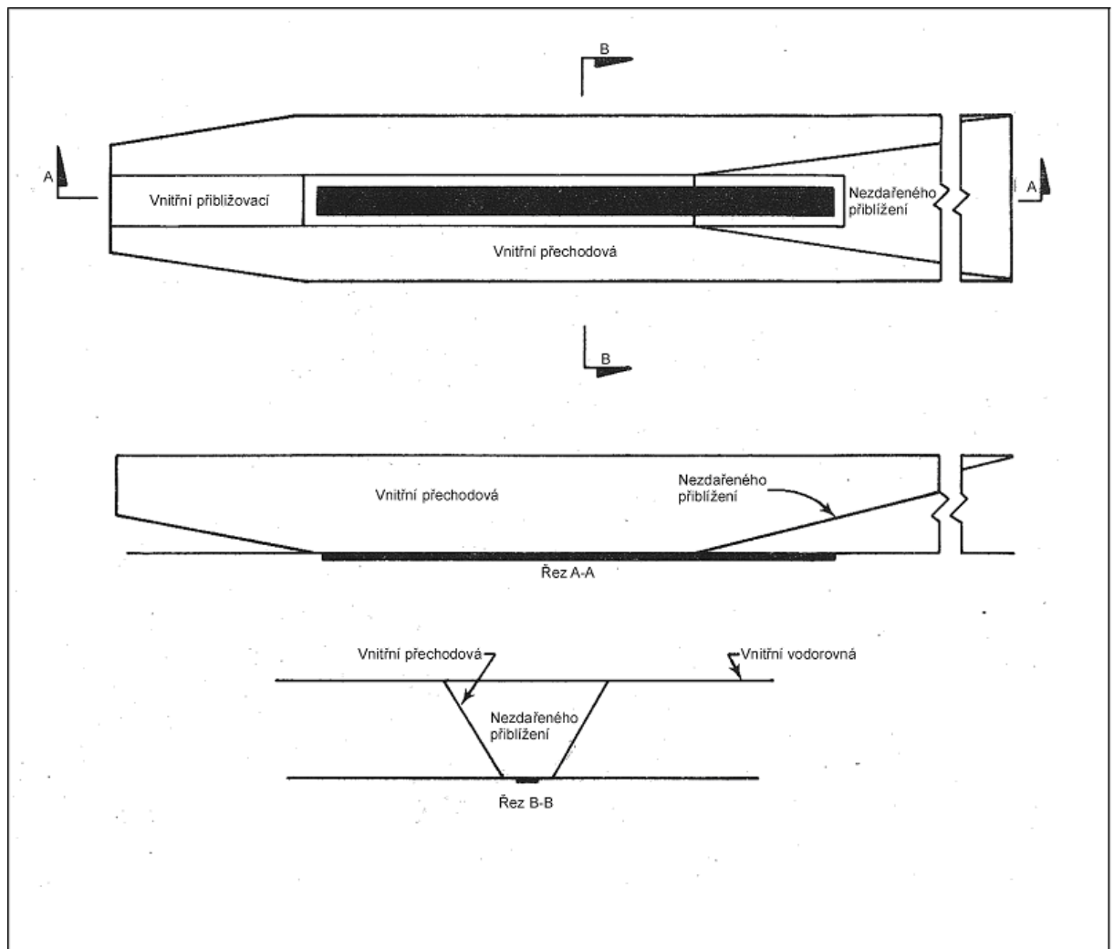
Obr. 4-2 Vnitřní přibližovací a vnitřní přechodová překážková plocha a překážková plocha nezdařené přiblížení
